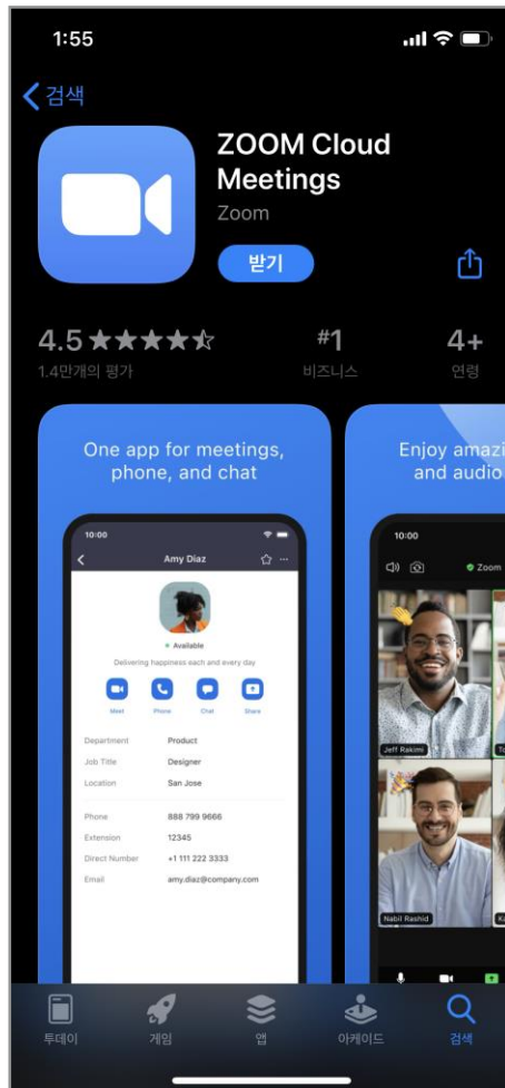
앱스토어 (IOS)
