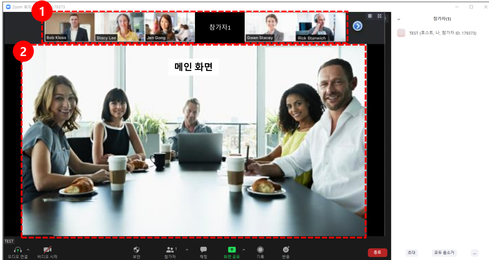
참가자 화면
