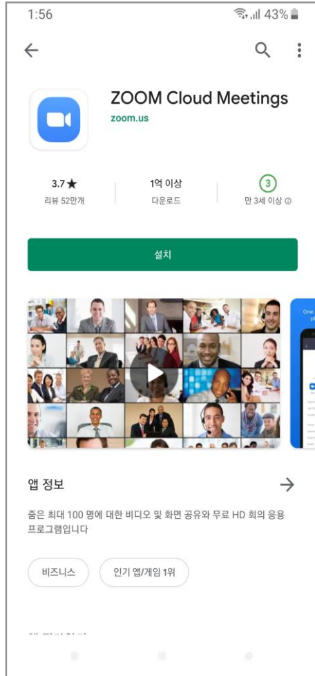
플레이스토어 (안드로이드)
